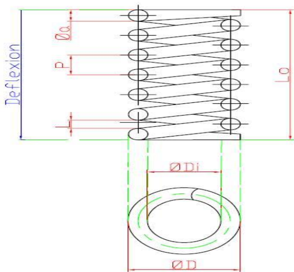
Grafico Dimensional Resorte Helicoidal
